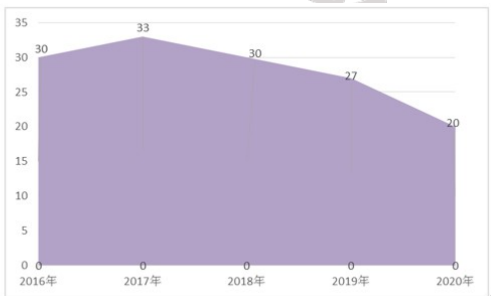
图 14 2016—2020 年中山 PM 2.5 浓度 (单位: 微克/立方米)
